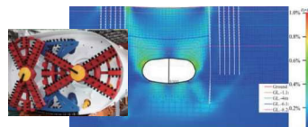
FEMtij-2Dを用いた矩形シールド掘進時の地盤等の変形挙動解析結果
