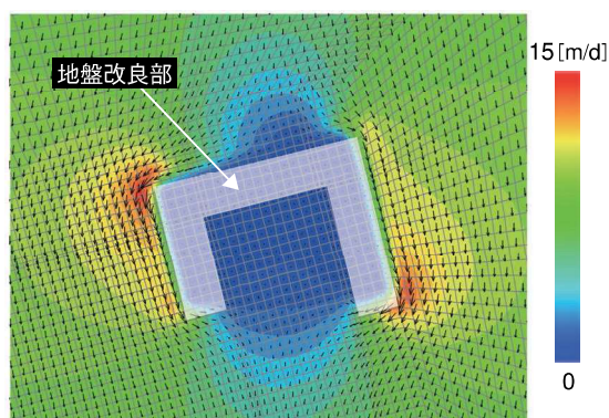
地下水流を地盤改良により遮水した際の地盤改良体付近の地下水流速分布
