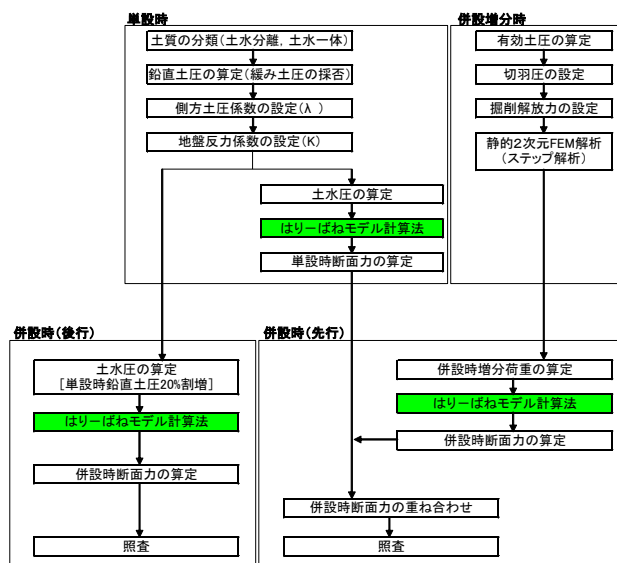
図-3 常時設計検討フロー 2)
