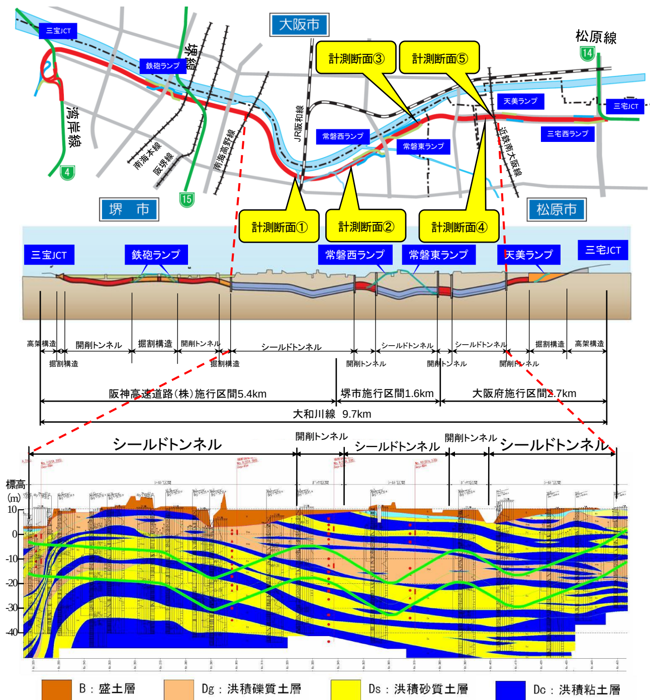
図-2 大和川線トンネル構造、事業区分、およびシールドトンネル区間の土質縦断面図
