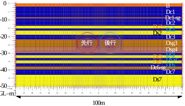
図-13 有限要素メッシュ図
