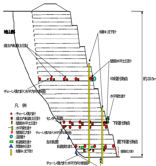
図-7 斜面形状と概略的計器設置図
