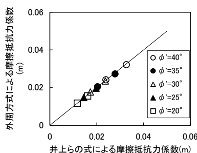
図-3 井上らの式と外周方式
