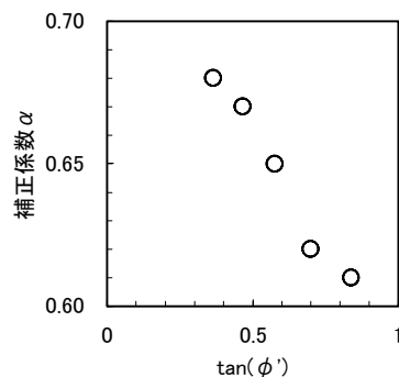
図-4 内部摩擦角と補正係数 \alpha
