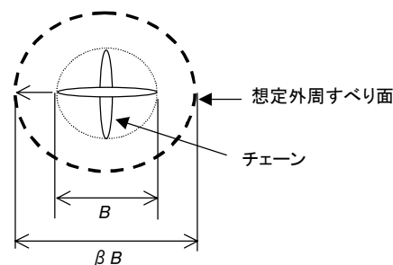
図-2 外周方式モデル
