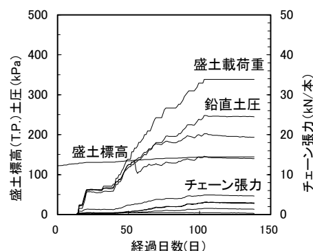
図-9 盛土に伴うチェーン張力
