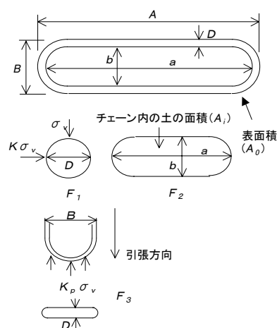
図-1 井上らのチェーン抵抗モデル
