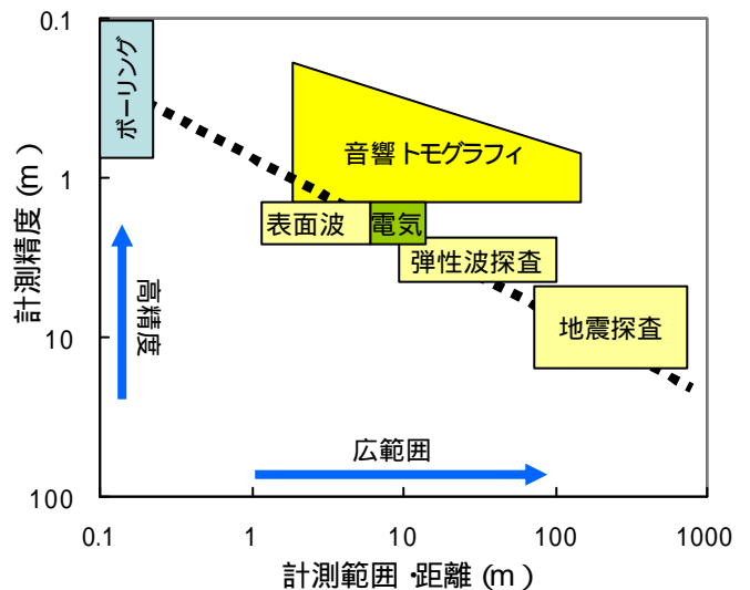
図-1 既存の探査手法との違い
