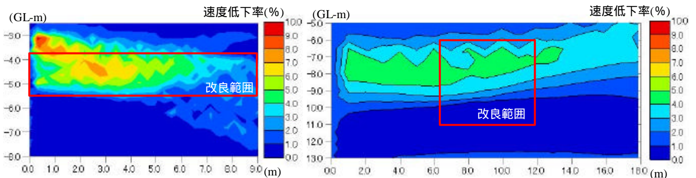
図-5 地盤改良直後の P 波速度低下率分布
