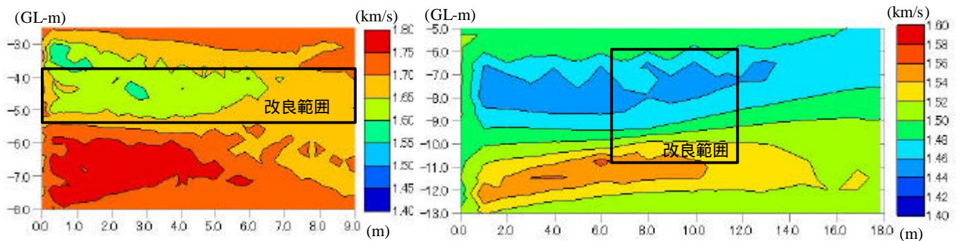
図-3 地盤改良直後の P 波速度分布
