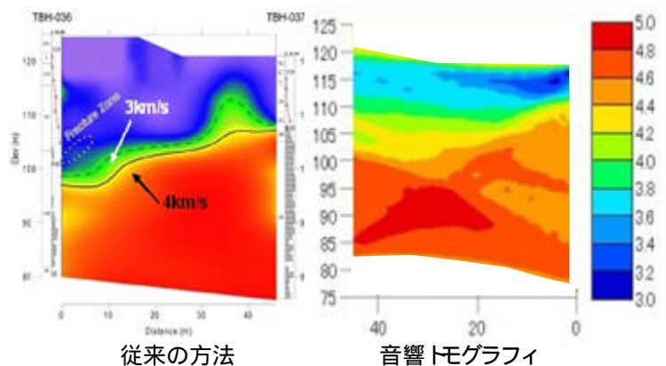
図-2 P 波速度の対比
